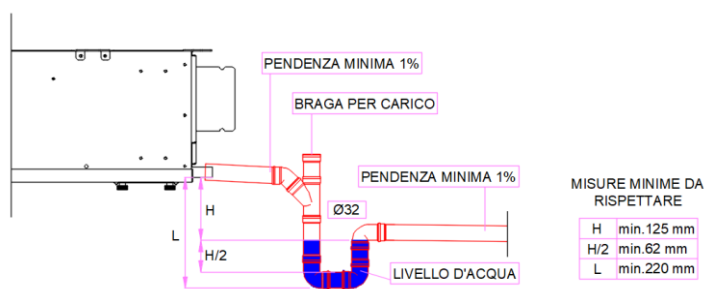
Allacciamento scarico condensa
